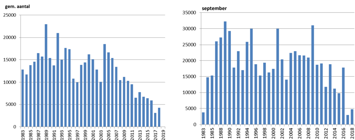
Figuur 1: Gemiddeld aantal water- en roofvogels per telling in het Natura-2000 reservaat. Tellingen in januari waarbij het Markiezaatsmeer grotendeels was dichtgevroren (1987, 1997, 2010) zijn niet meegeteld. Rechts: de aantallen die in september werden geteld.
